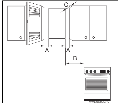
Fig. 20 Distâncias mínimas
