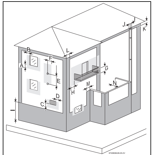
Fig. 21 Distâncias mínimas a pontos de exaustão
