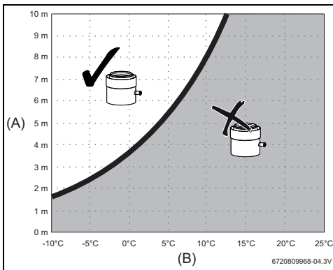
Fig. 4 Condutas concêntricas
