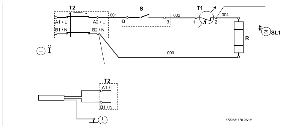
Fig. 5 Esquema de ligação
