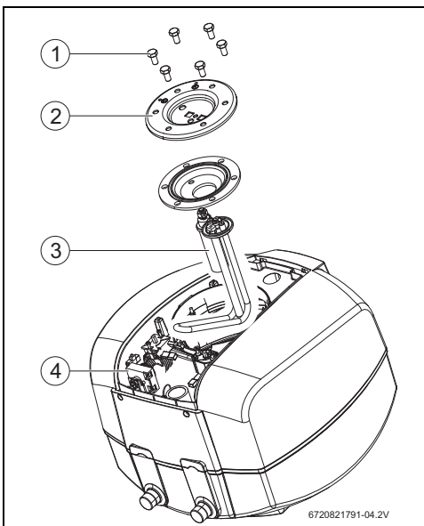
Fig. 14 Acesso e identificação dos componentes internos
