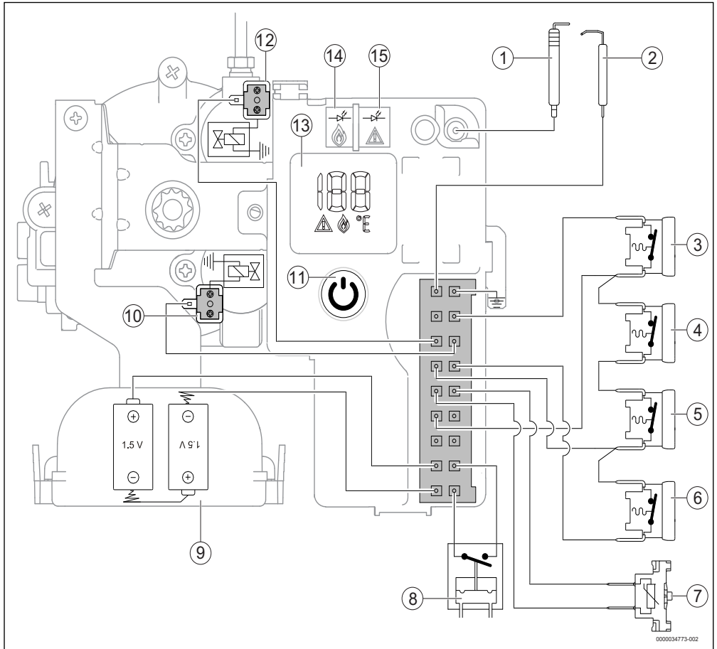
Fig. 26 Esquema elétrico
