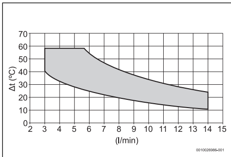
Fig. 28 Modelo 14 litros
