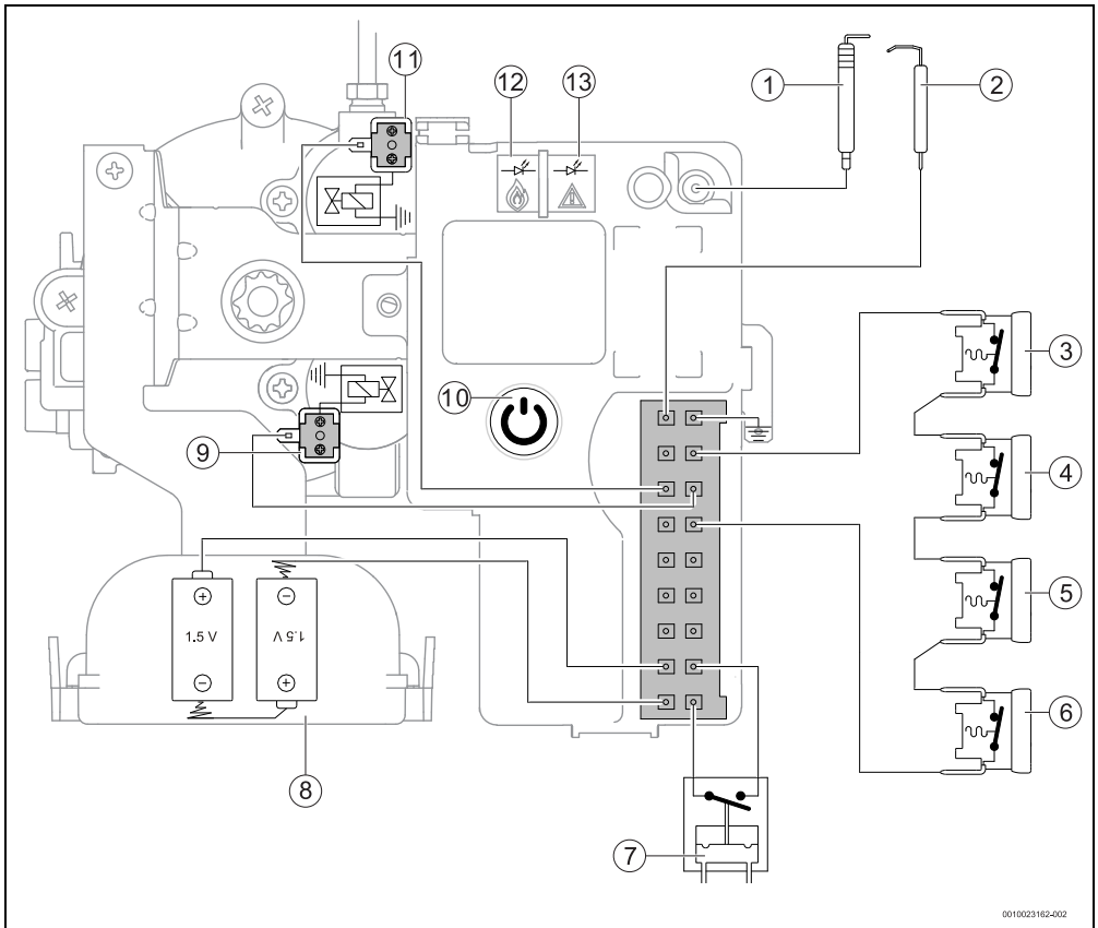
Fig. 25 Esquema elétrico
