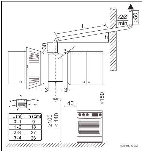
Fig. 11 Distâncias mínimas (cm)
