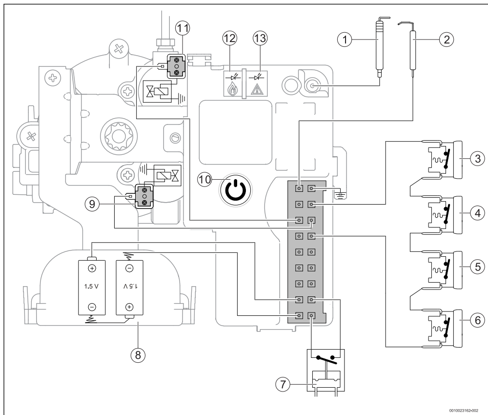
Fig. 26 Esquema elétrico
